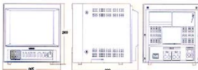
Dimensiones externas ( mm )
